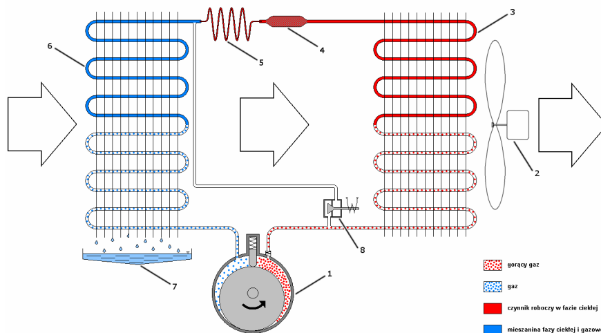
Zasada działania sprężarkowego osuszacza kondensacyjnego w fazie normalnej pracy: 1 – sprężarka, 2 – wentylator, 3 – skraplacz, 4 – filtr (odwadniacz), 5 – organ dławiący, 6 – parownik, 7 – zbiornik kondensatu (skroplin)
