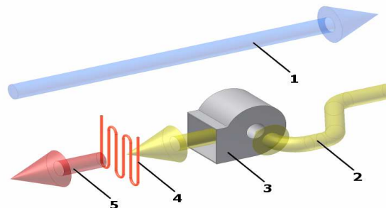
Osuszanie przez wentylację i ogrzewanie: 1 - powietrze wyrzucane na zewnątrz, 2 - powietrze zasysane z zewnątrz, 3 - wentylator, 4 - nagrzewnica, 5 - ogrzane powietrze
