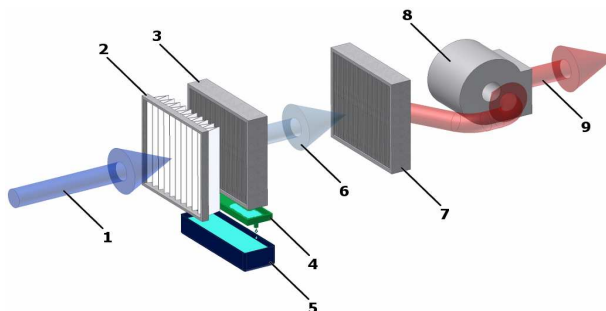
Osuszanie kondensacyjne: 1 – wilgotne powietrze, 2 - filtr, 3 - parownik, 4 – taca oleikowa, 5 – zbiornik kondensatu, 6 – osuszone i schłodzone powietrze, 7 – skraplacz, 8 – wentylator, 9 – osuszone i ogrzane powietrze
